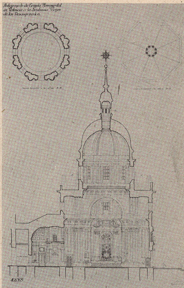
Anteproyecto de Templo Monumental, en Valencia, a la Santísima Virgen de los Desamparados. Arquitecto, J. Fernández Golfín.
